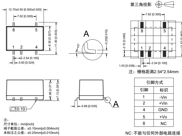
封装尺寸图
